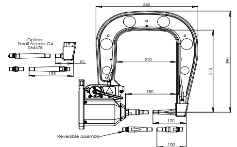
G14 - 080942 8 bar / 550 daN
