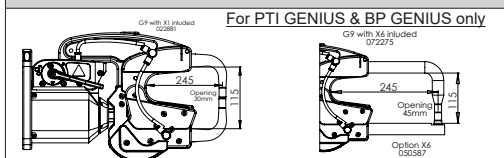
G9_X1 - 022881 8 bar / 550 daN
