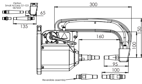
G1 - 022768 8 bar / 550 daN
