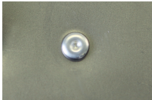
RÉSULTAT DE POSE D'UN RIVET FLOW-FORM
