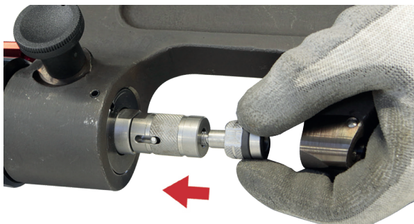
Supporto punzone / mandrino
